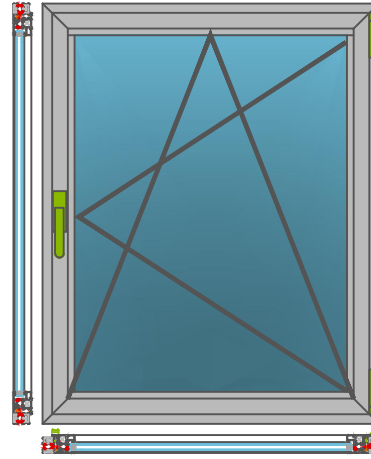
Test Numunesinin Ebatları Test Sample's Dimensions
